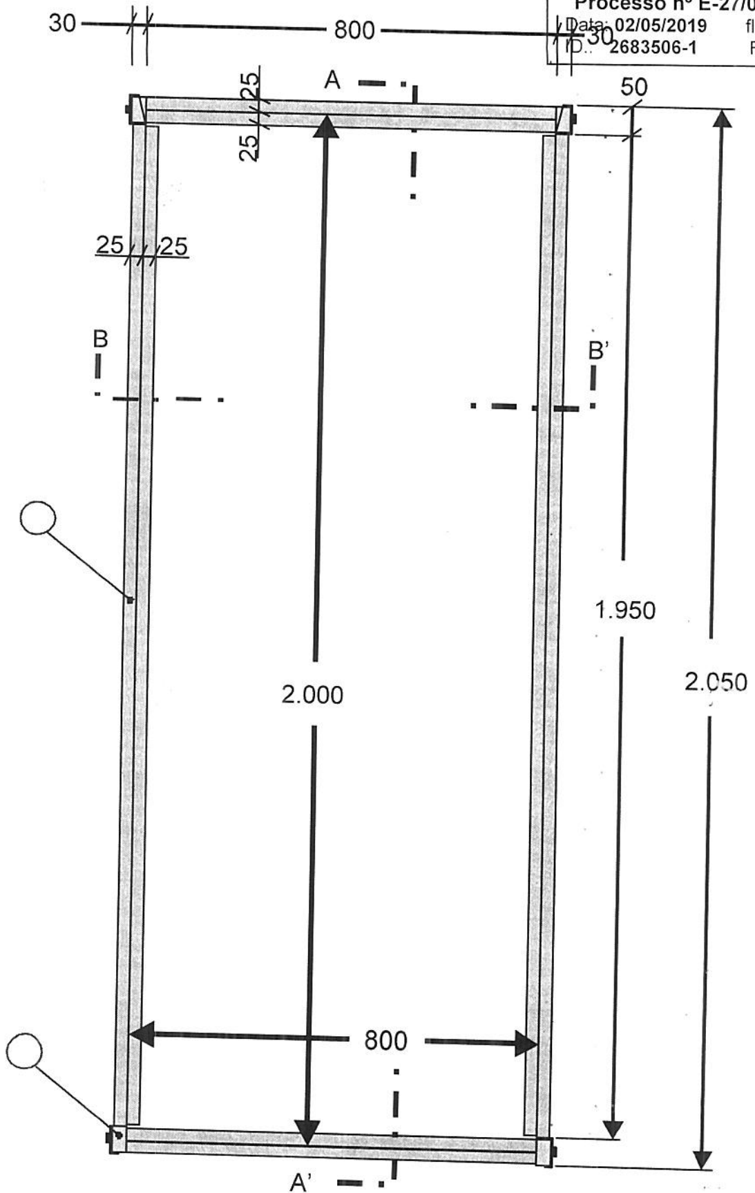
Figura 2 – Vista de topo ( medidas em milímetros )
