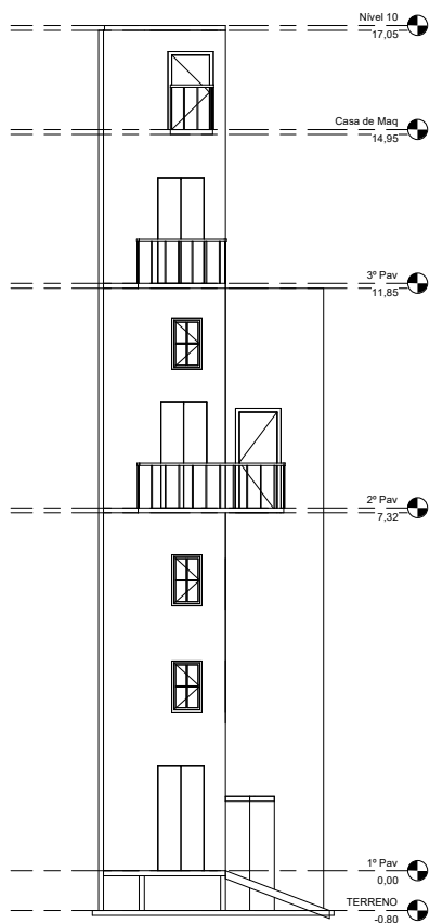
5 Corte 1 1 : 50 Corte Frontal
